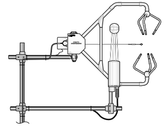
CSAT3 and CS7500
